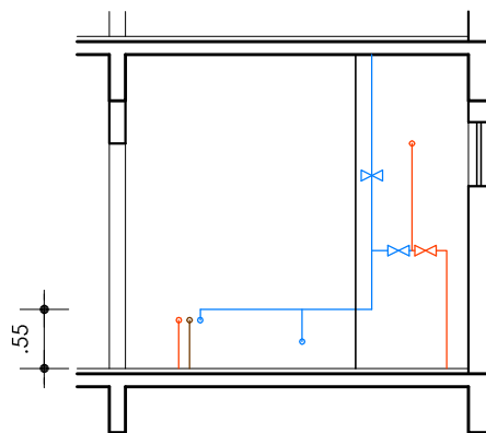
Banheiro Social
